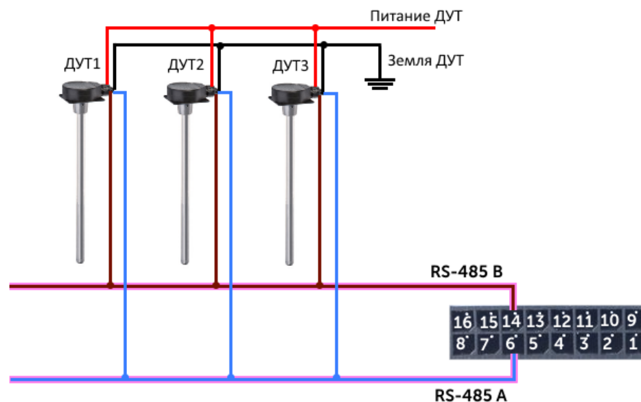
Рис. 4.5. Схема подключения датчиков уровня топлива к шине RS-485.
