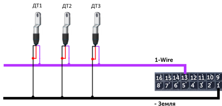
Рис. 4.1. Схема подключения датчиков температуры к шине 1-Wire.
