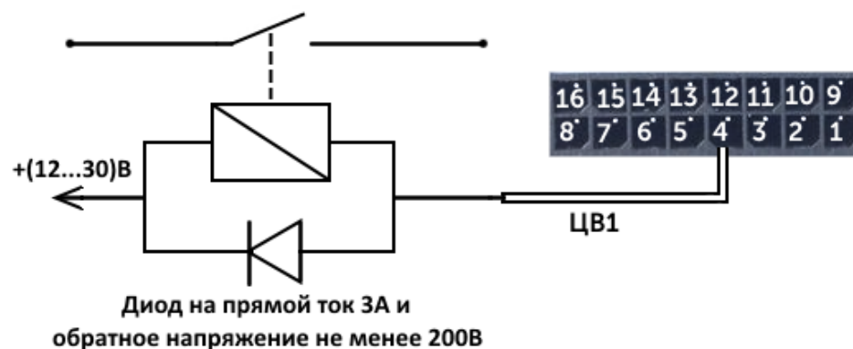
Рис. 4.6. Схема подключения реле на Цифровой выход 1.
