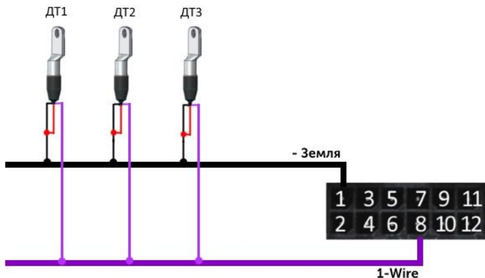
Рис. 4.1. Схема подключения датчиков температуры к шине 1-Wire.
