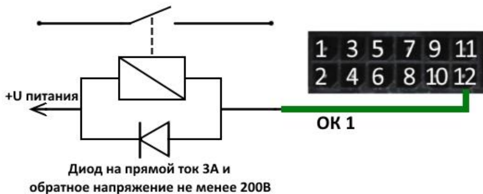
Рис. 4.6. Схема подключения реле на выход «открытый коллектор» 1.
