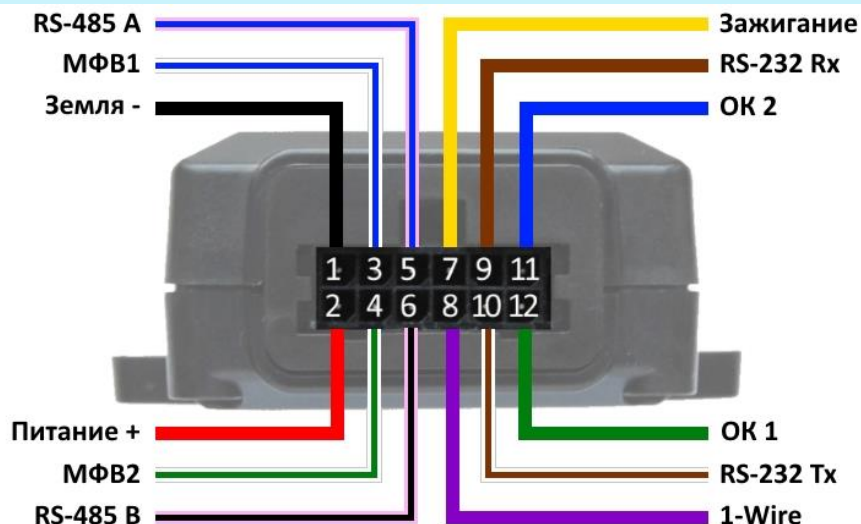
Рис. 3.1. Расположение контактов в разъёме.
